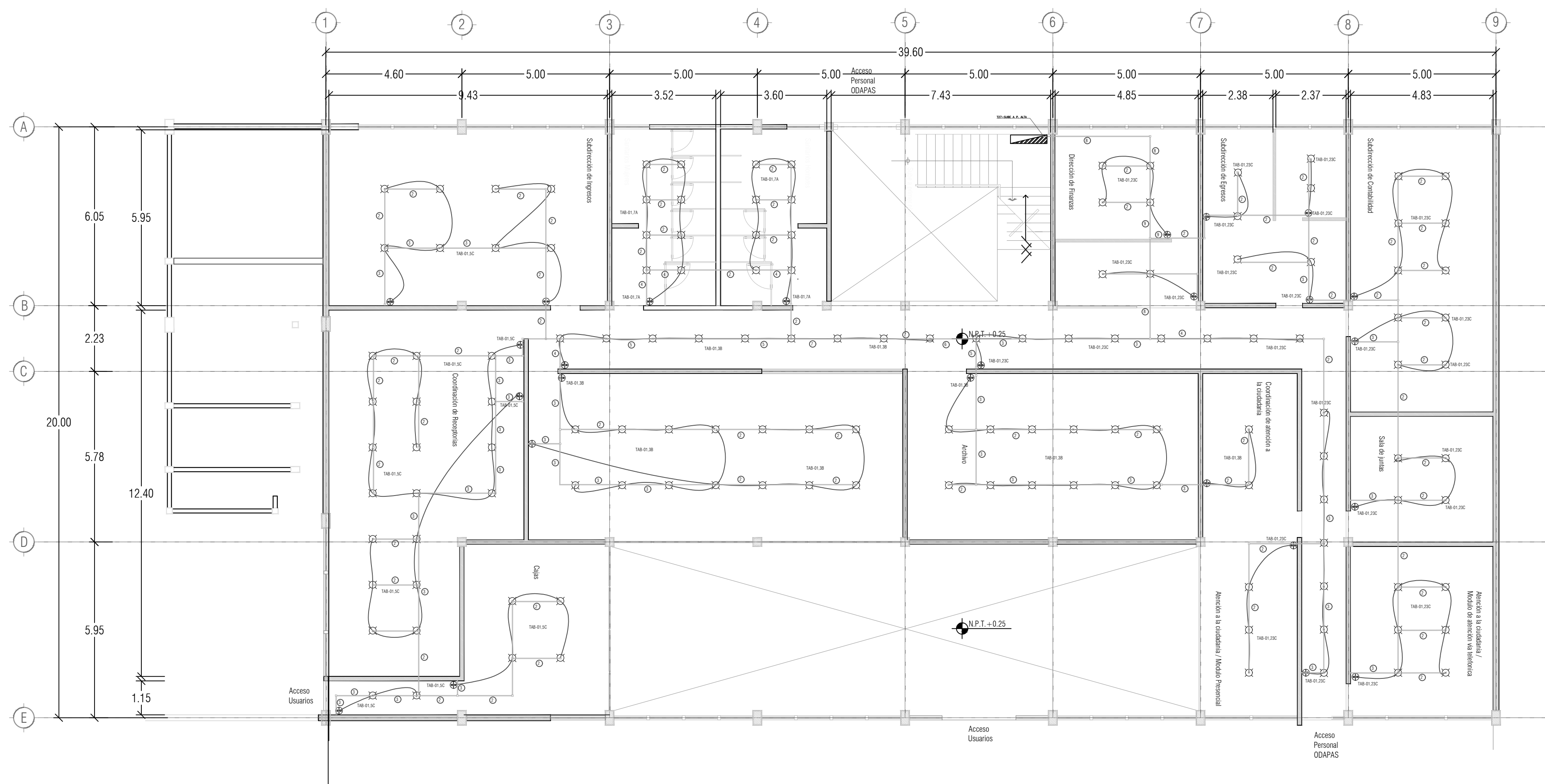
PLANTA BAJA
