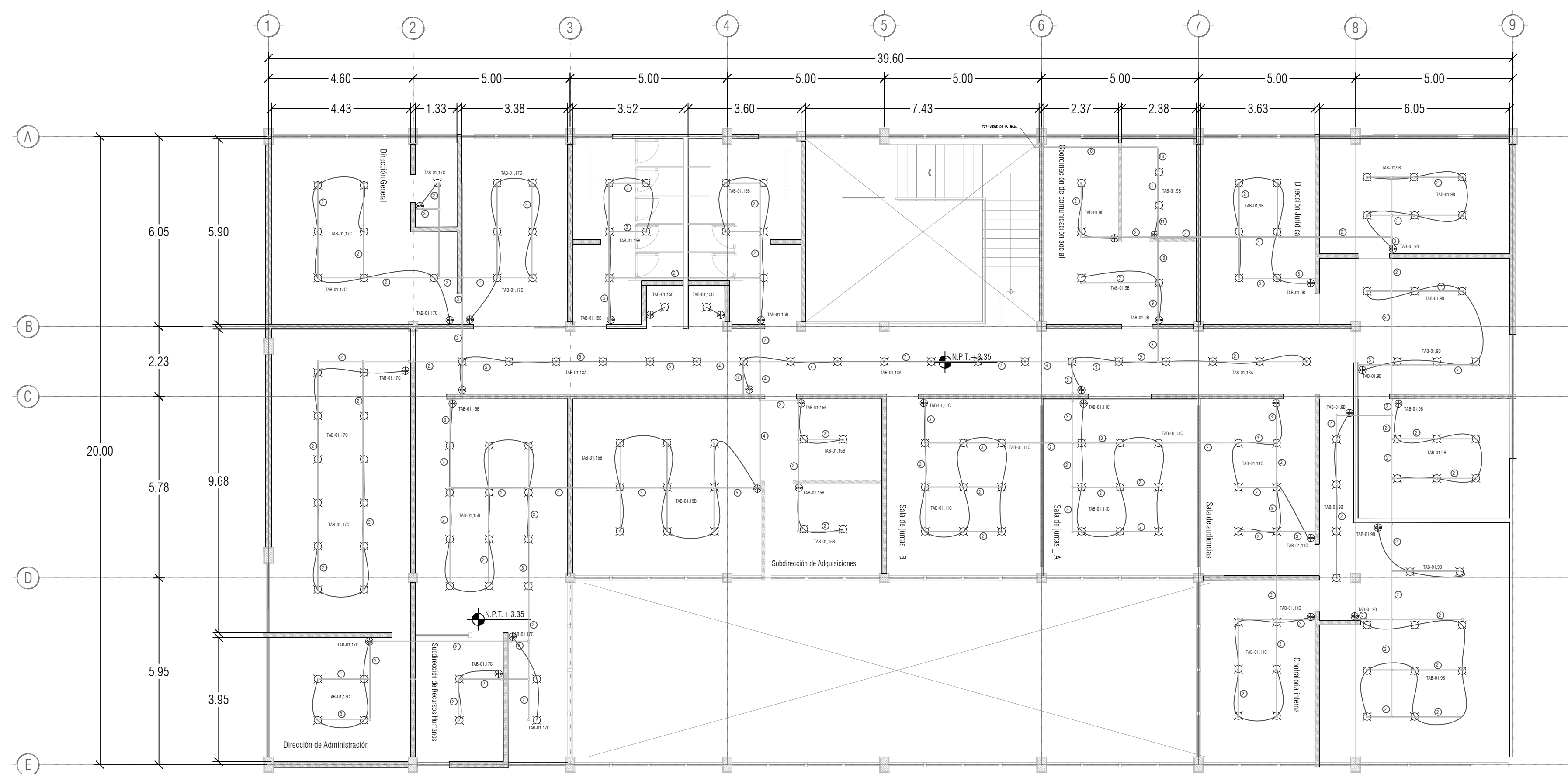
PLANTA ALTA
